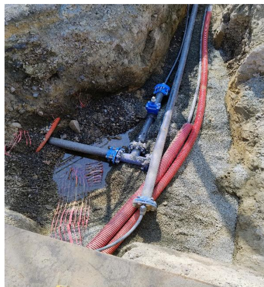
Photos de la desserte du lotissement de Cavan
